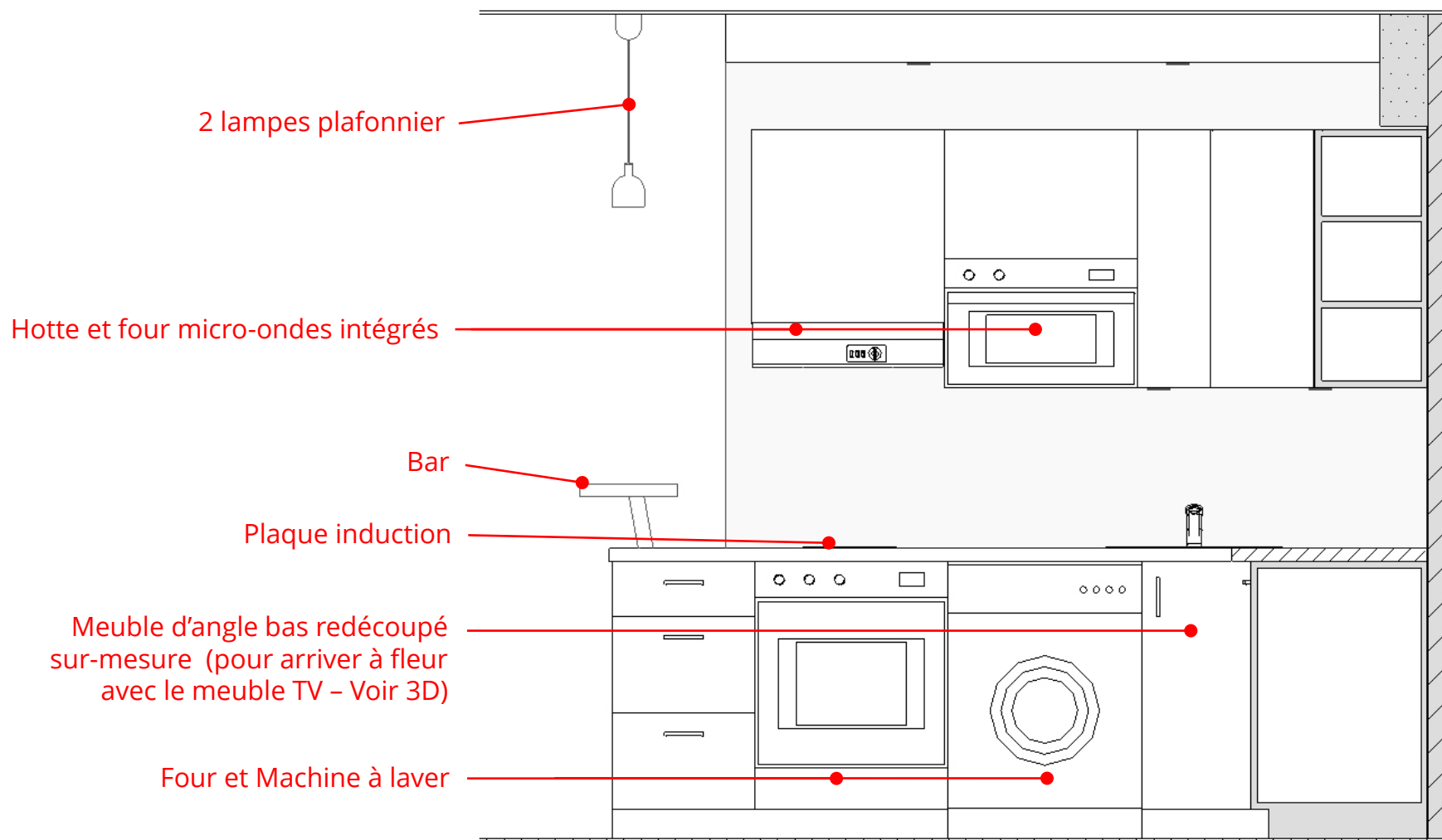
Plan d'élévation cuisine (vue depuis l'entrée)
